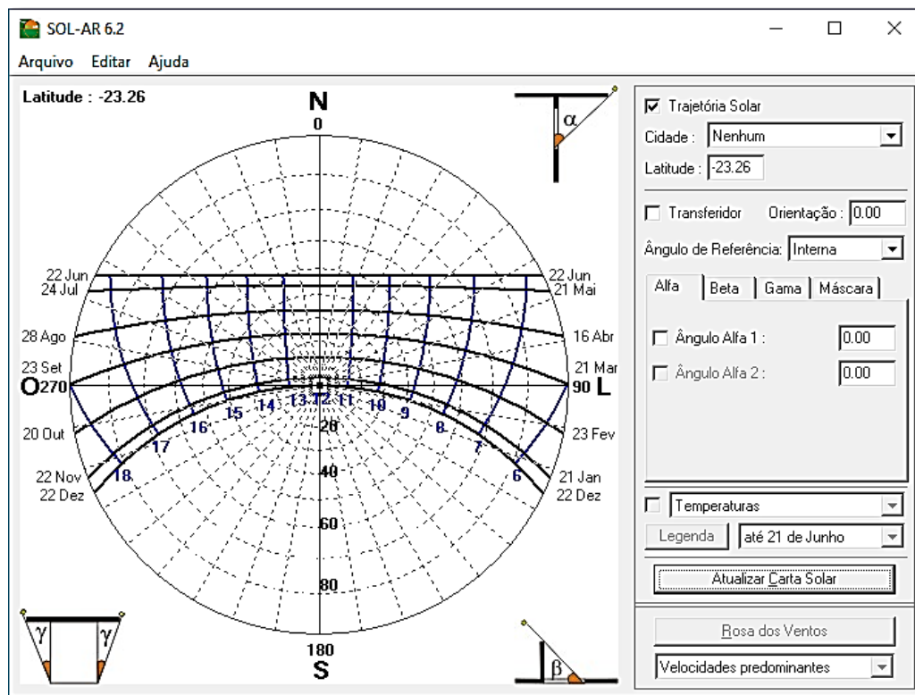
Gráfico 7 - Mapa solar do povoado de Aqui – Latitude, 23^\circ 26' 22'' .
